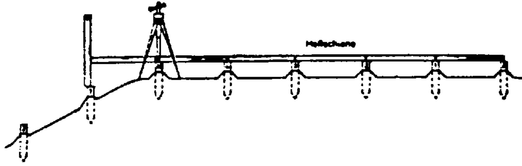
(شكل ١٤) طريقة القياس
